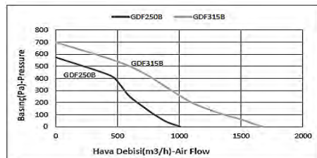
GDF 250-315
