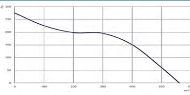
GKAF 160
