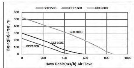
GDF150-160-200
