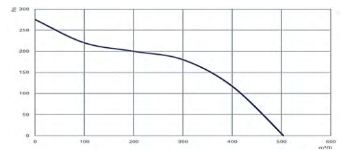
GKAF 250
