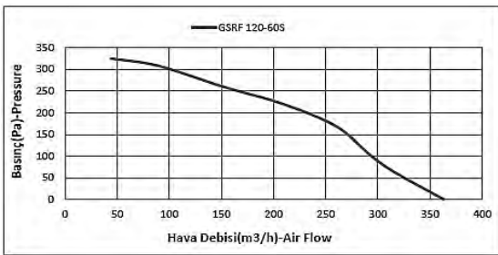
GSRF 120-60
