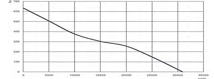
GBSK 900-5-40
