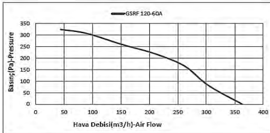
GSRFA 120-60
