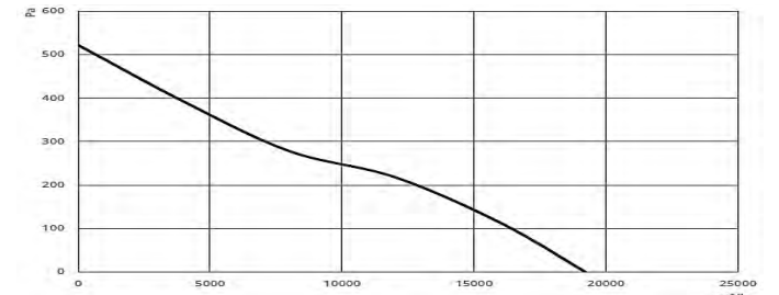
GBSK 800-5-35
