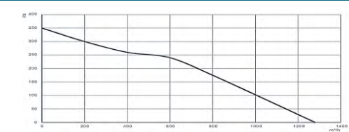
GKAF 250
