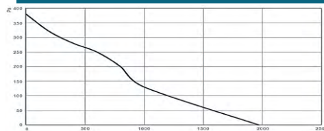
GKAF 200
