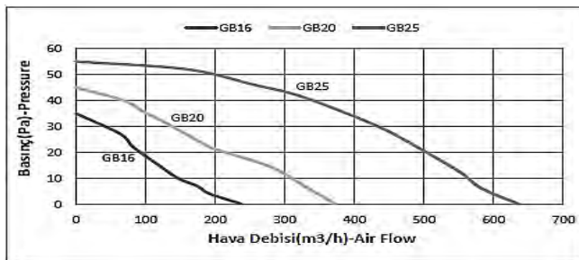
GB16-20-25
