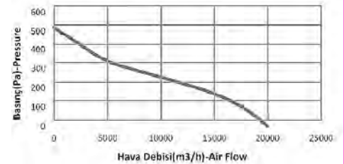
GAV 1000 T
