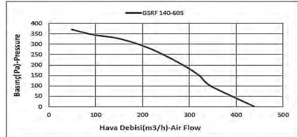
GSRF 140-60
