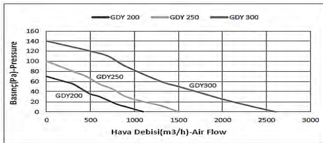
GDY200-250-300
