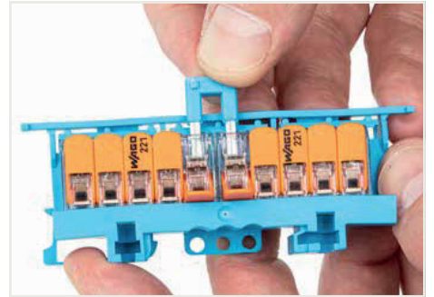
Köprüyü açık kelepçelemeye birimlerinden çıkarın.
