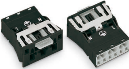
Kendinden topraklı ankastre modül. Yuvasına oturttuğunuz anda şaseye toprak bağlantısı doğrudan uygulanır.
