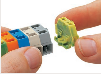
Modüler klemenslerin grup montajı.
