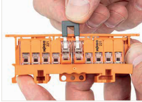
Köprü kilitleme işlevi olmadan açık kenetleme birimlerine takın.
