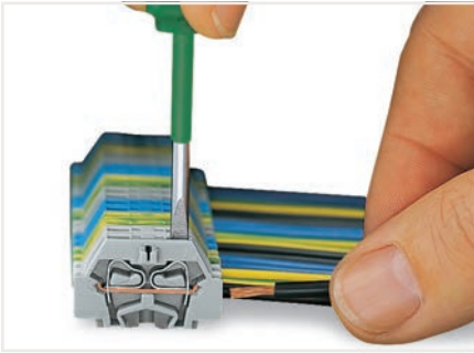
Bir iletken yerleştirme.
