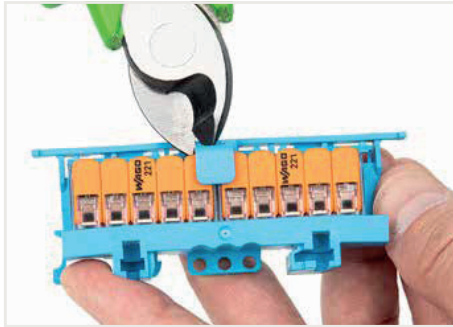
Köprüyü çıkarmak için kilitleme mekanizmasını çıkarın.
