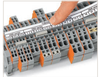
Bir şerit etiketi, etiket yuvasına takma.
