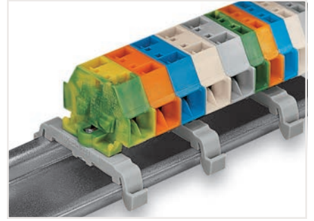
DIN-35 rayı üzerinde montaj flanşlı klemens dizisi
