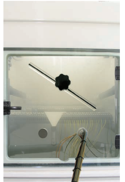
Tuzlu su testi
