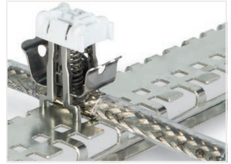
Ekran sıkıştırma modül kontakları ekran iletkeni ve özel yanıklı DIN rayı (790-145). Lütfen rayın altındaki ara modülü (790-144) kullanın.
