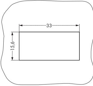
Ankastre için açılacak yuva ölçüleri
