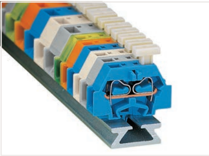
Bir tarafta basma butonlu klemens şeridi
