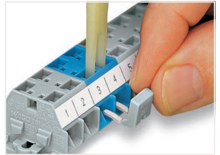
Tarak tarzı köprü ile ortaklaştırma.
