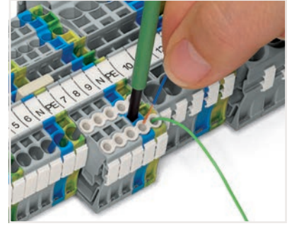
Yalıtım durdurucusuna bir iletken takın.
