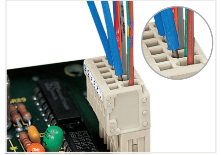
1 mm Ø test pini (Ürün No. 735-500) ile test, kontakla dokununuz.
