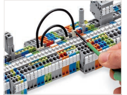
Tamamen yerleştirilene kadar tel köprüyü aşağı doğru itin. Yeniden kablolama yapmak için köprüyü bir el aletiyle çıkarın.
