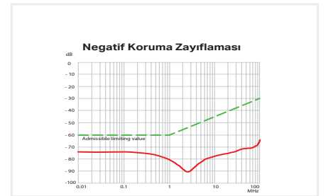
Blendaj bağlantı sistemi oldukça etkilidir çünkü sıkıştırma ünitesi kabloların blendajsız kısmına çok yaklaştırılabilir.
