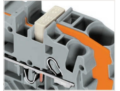
İndirgeme köprüleri ile köprüleme.
