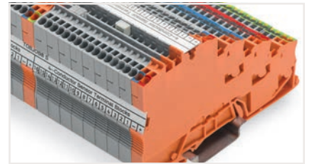
Şerit etiketler ile etiketleme (2009-110) (üstten veya yandan)
