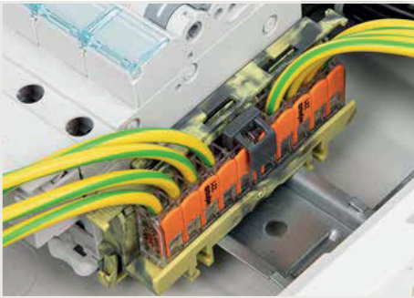
Kilitlelenebilir köprü, eklemeye konektörlerine takılır.
