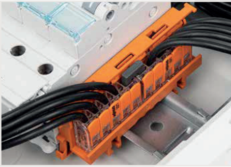
N ve PE (toprak) dağıtımını köprü ile genişletme
