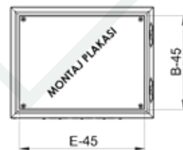
İÇ GÖRÜNÜŞ
